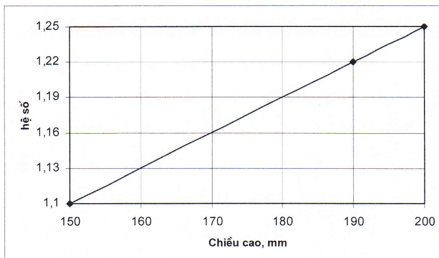
Biểu đồ 1 : Xác định hệ số mẫu có chiều rộng 150 mm, chiều cao 190 mm
